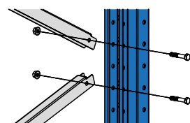
Stoßpunkt Rahmenfachwerk
