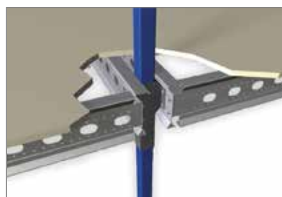
Stützen
