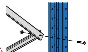
Kreuzungspunkt Rahmenfachwerk
